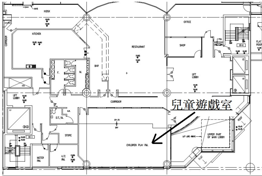
工程地點平面圖
