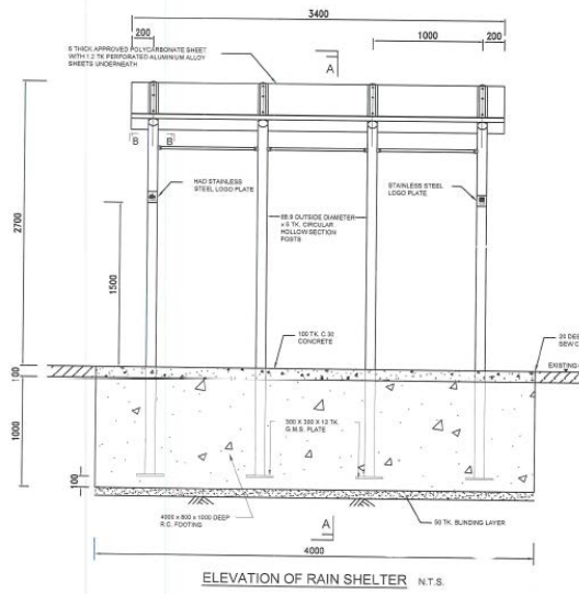
避雨亭設計圖
